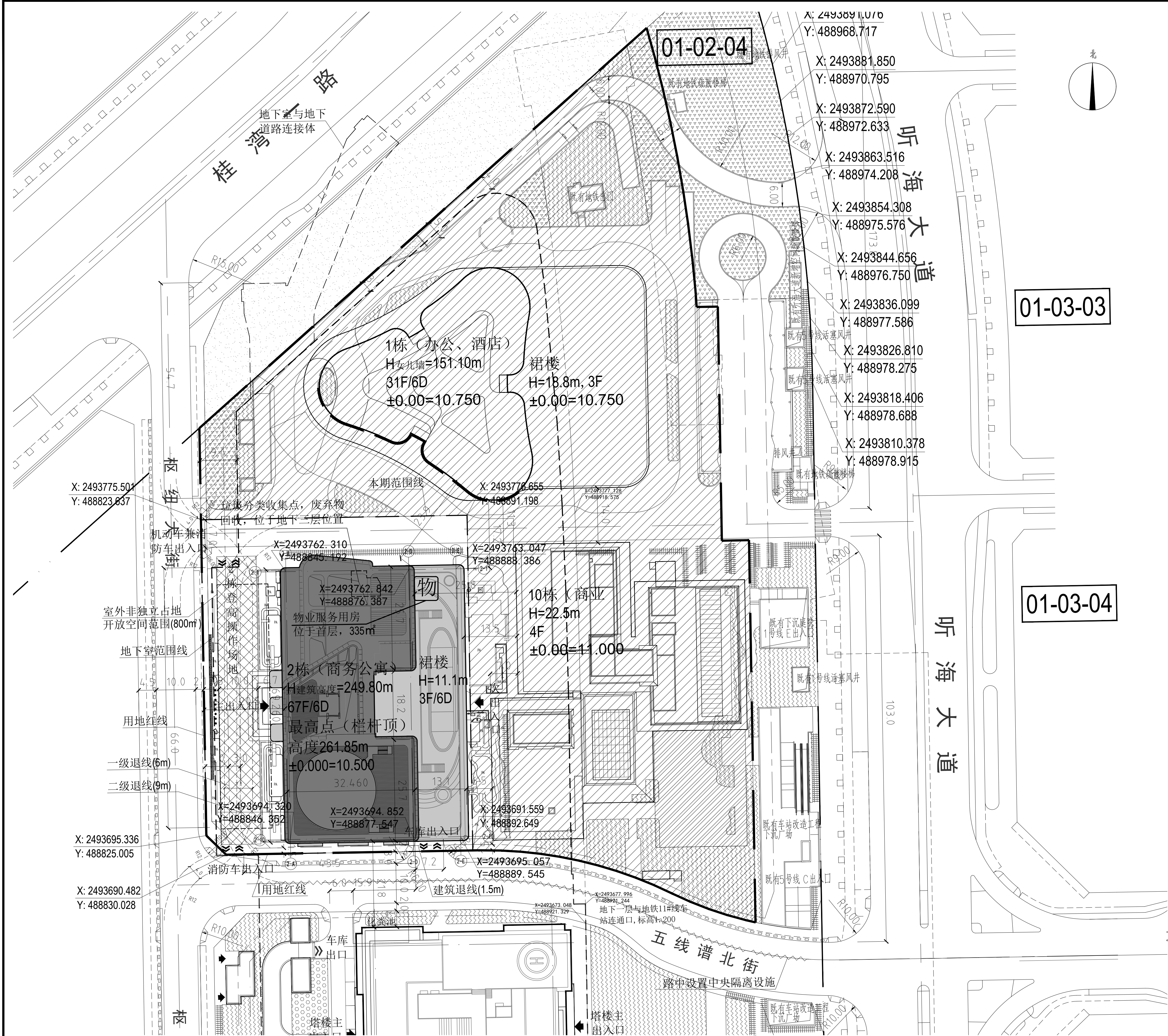
2栋总平面图 1:500
