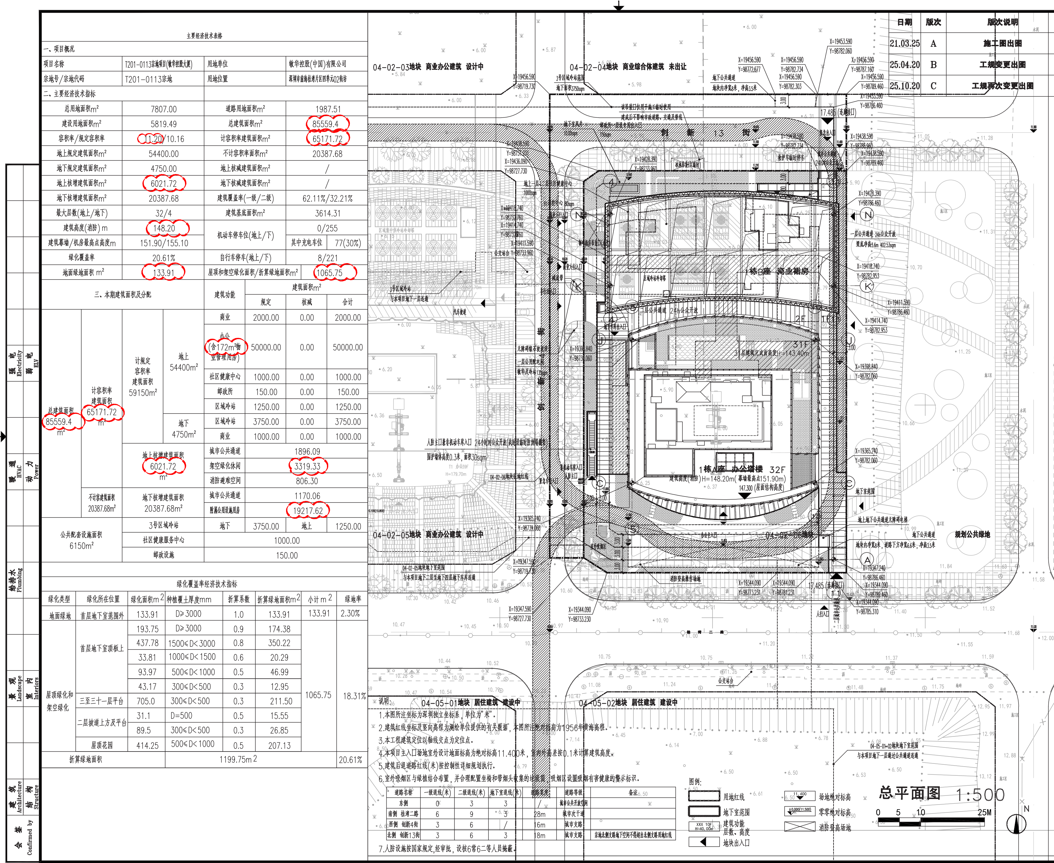
修改后总平面图
