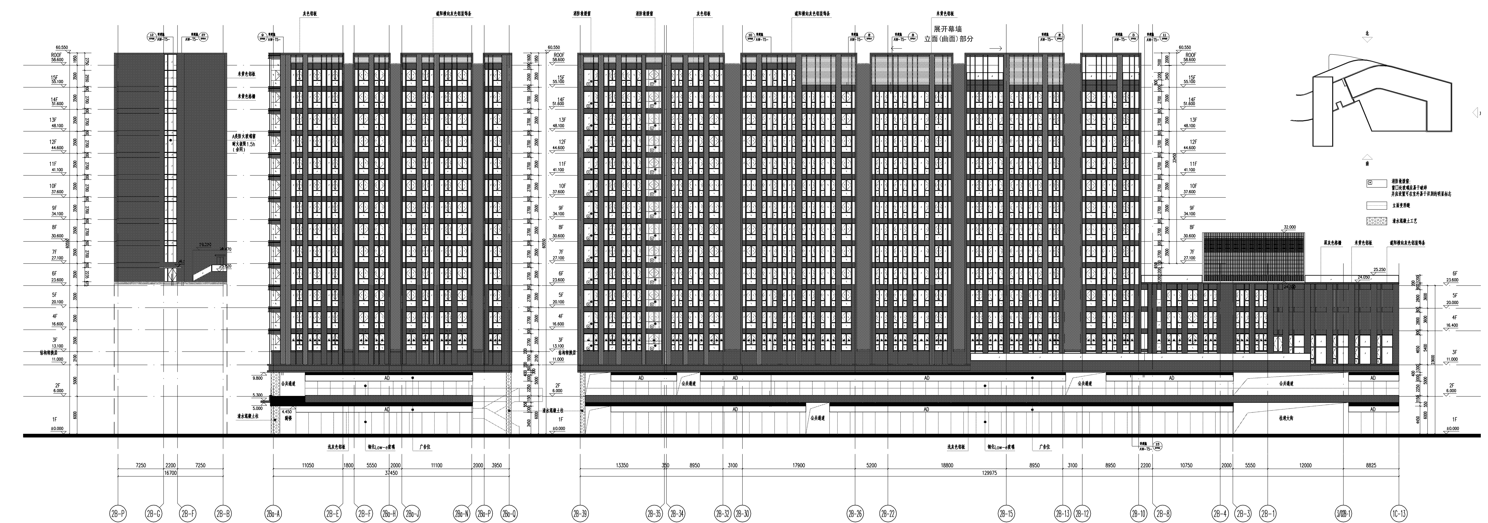
2B-P 轴 ~2B-B 轴立面图
