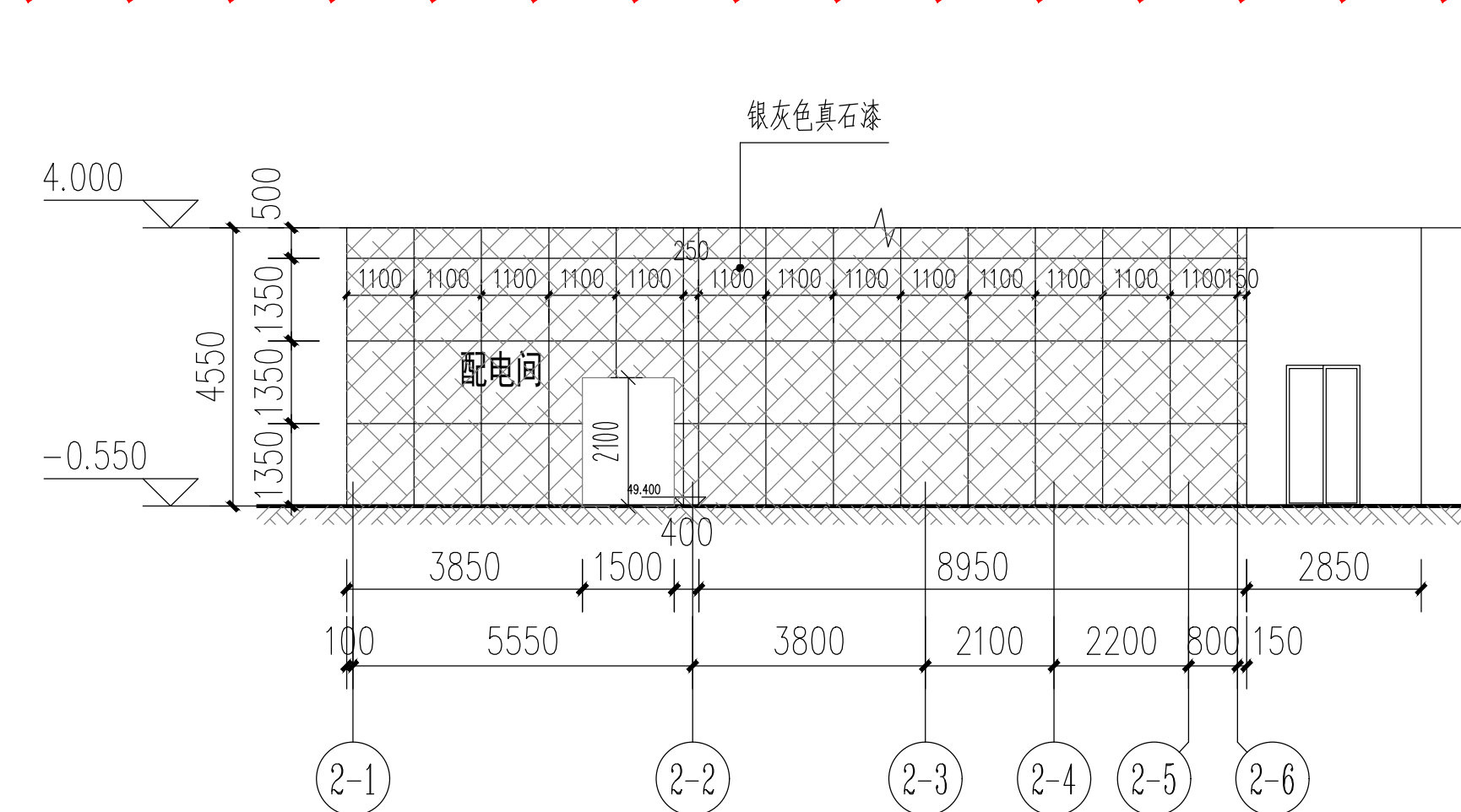
候车室东南面立面图 1:150
