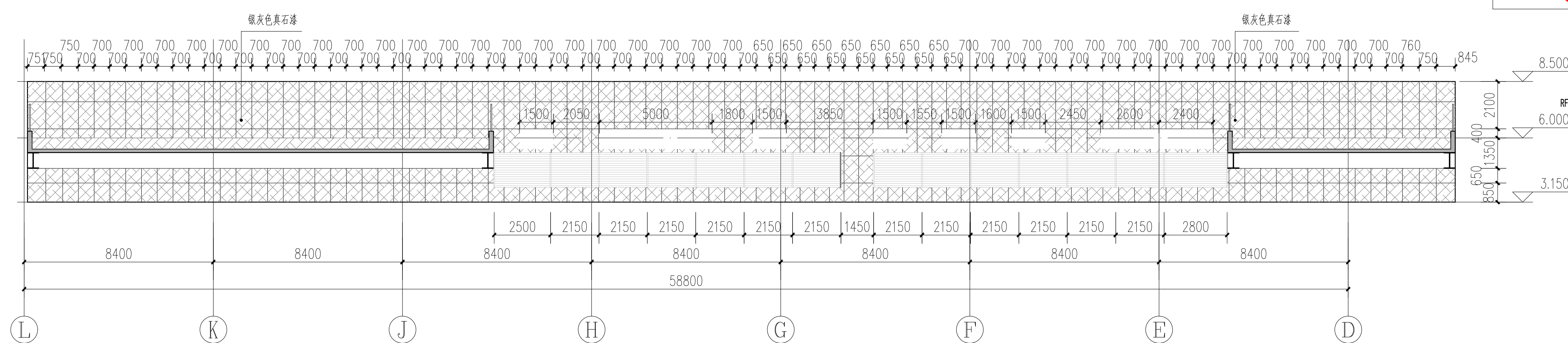
站务用房④~⑤轴立面图 1:150
