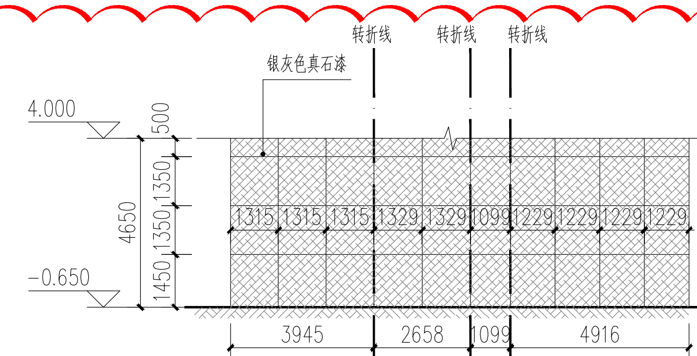
监控室展开立面图 1:150
