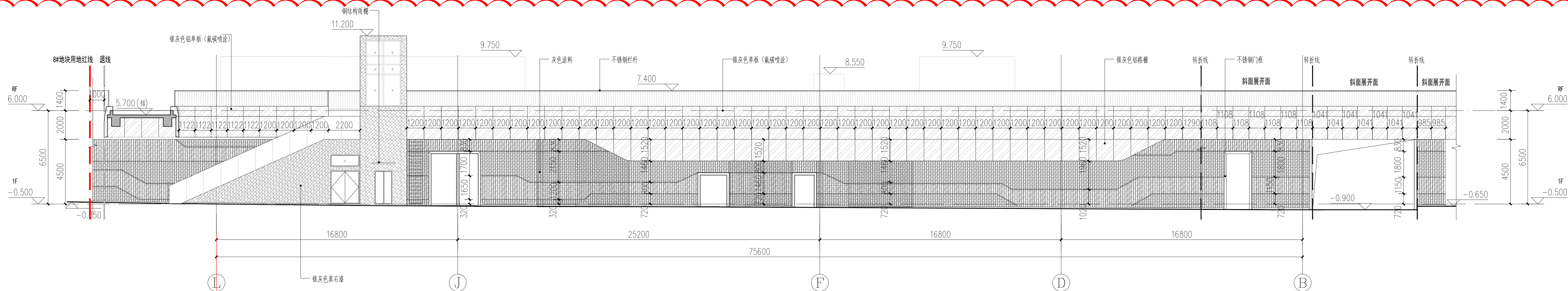
公交首末站①~②轴立面图 1:150
