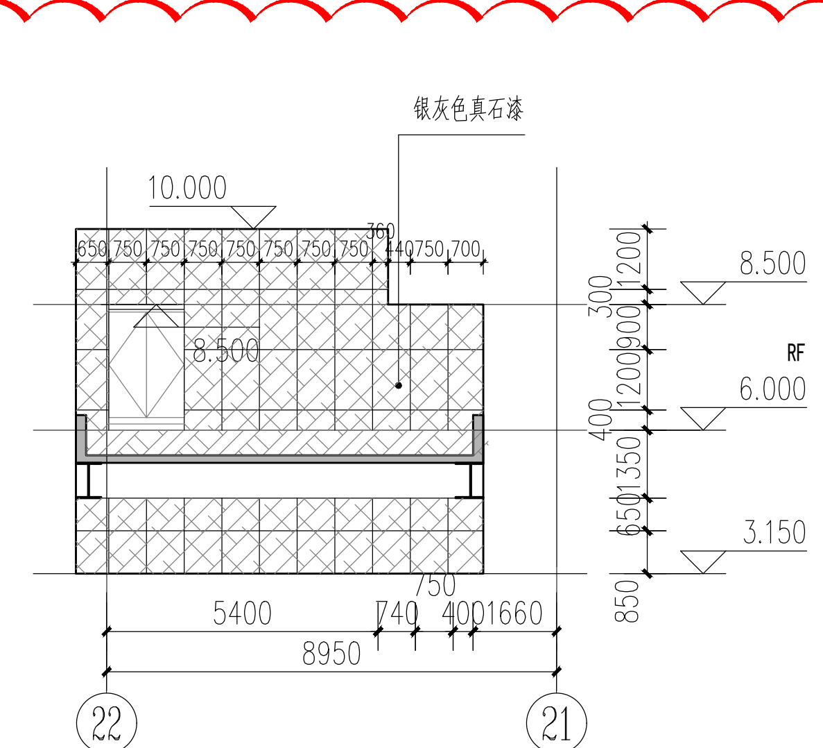
站务用房②②~②①轴立面图 1:150
