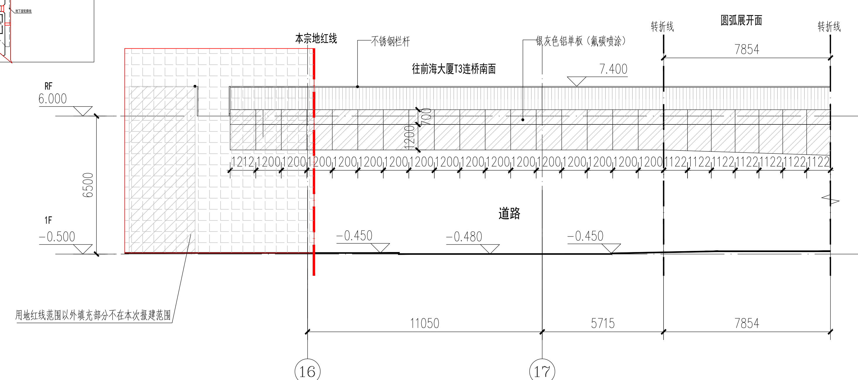
连桥 ⑬~⑰轴立面图 1:150
