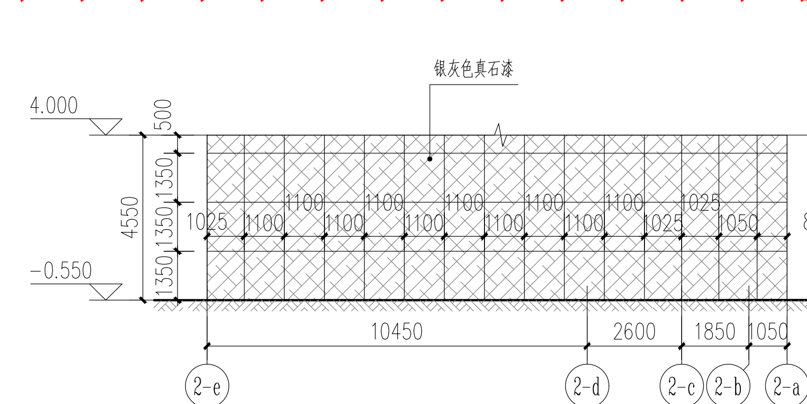
候车室西南面立面图 1:150
