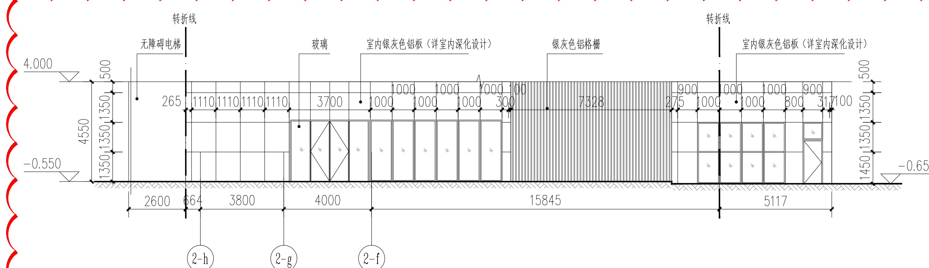
候车室东北面展开立面图 1:150
